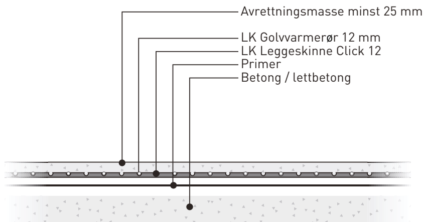
LK Leggeskinne Click 12 mot undergulv av betong eller lettbetong.
